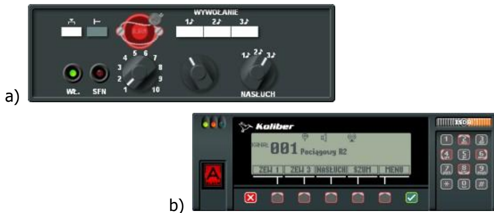
图 2.4.8 ISDR 中两种无线电接发设备 (其中：图 a 为拉德莫 (Radmor) 3006 型电台 图 b 为克利贝尔 (Koliber) 型电台)
