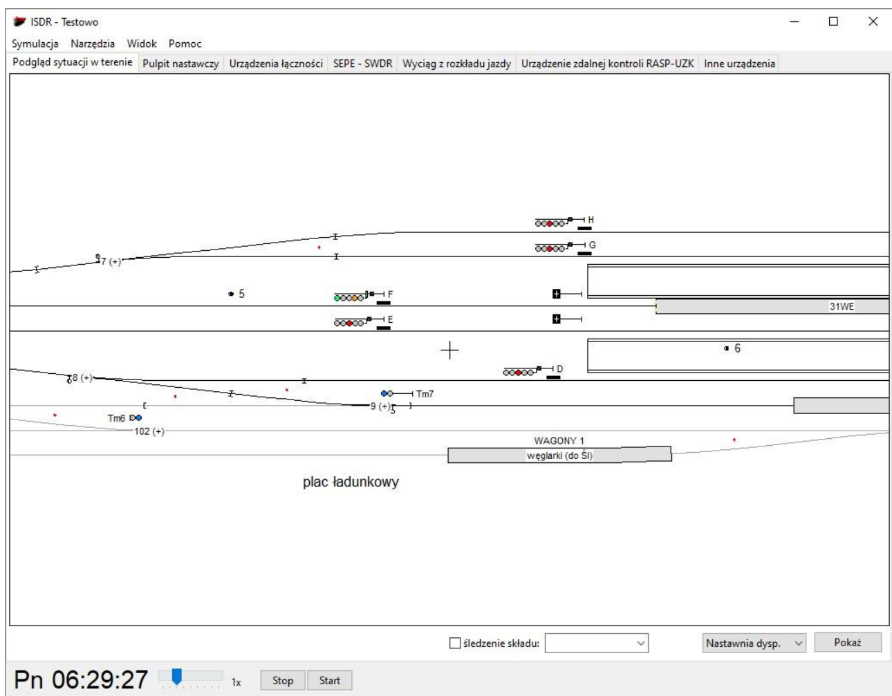
图 2.2.1 现场情况概览窗口
