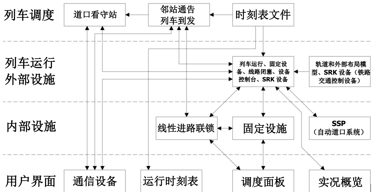
图 1.1 ISDR 模拟器架构简化图
