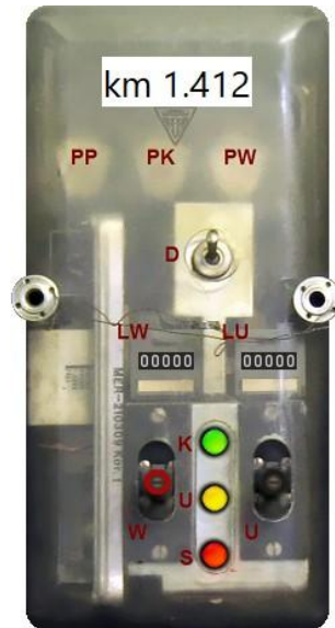
图 2.6.1 ERP-5 型远程控制设备
